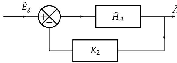
FIGURE 4 – Schéma bloc de l'asservissement d'accélération
