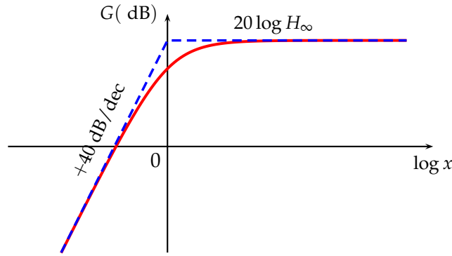
FIGURE 2 – Diagramme de BODE de |\underline{H}_A(jx)|
