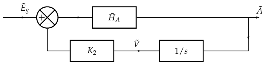
FIGURE 3 – Schéma bloc de l'asservissement de vitesse
