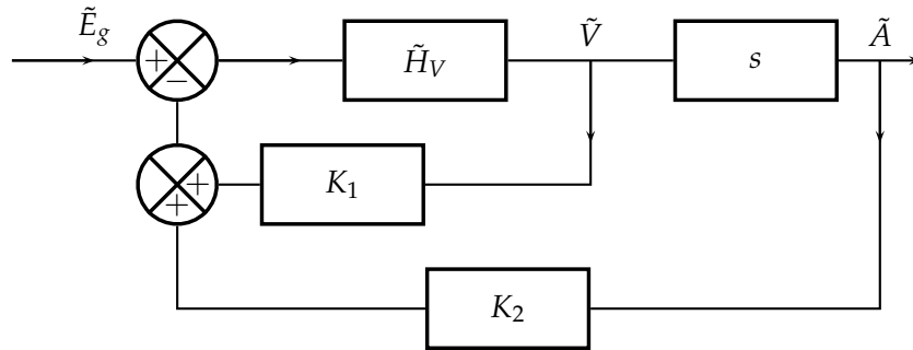
FIGURE 5 – Schéma bloc de l'asservissement mixte
